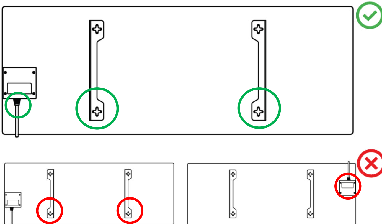
Obrázek 7 – Instalace držáků
