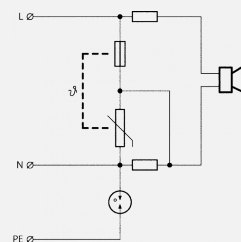
Schéma zapojení
