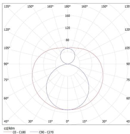
KANLUX S.A. (kat 26062) T8 LED GLASSv3 9W-NW / LDC (Polar)
