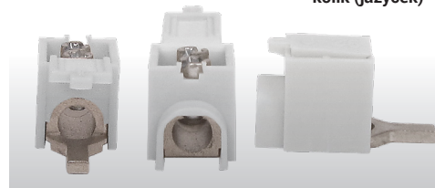
2 šrouby pro utažení vodiče (vhodné pro měděné vodiče do průřezu 25 mm 2 )
