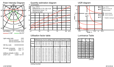
TCW060 1xTL-D58W HF
