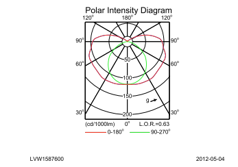
TCW060 1xTL-D58W HF
