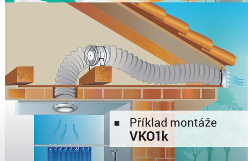
■ Příklad montáže VK01
