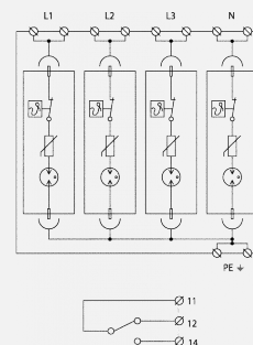
Schéma zapojení
